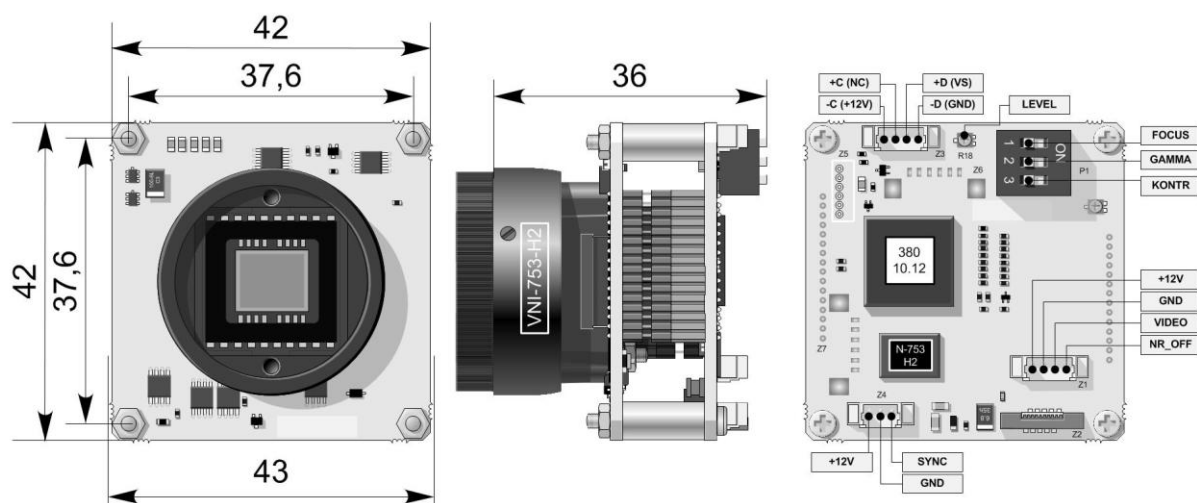
Рис.1. Камера VNI-753-H2-VS
